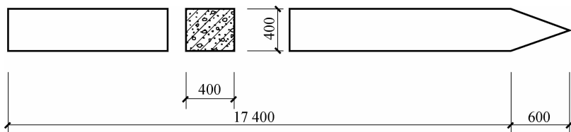
图 4-29 预制桩
