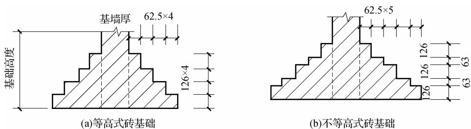
图 4-32 砖基础断面图
