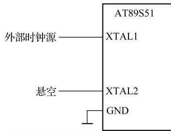
图 1-4 AT89S51 外部时钟方式的电路
