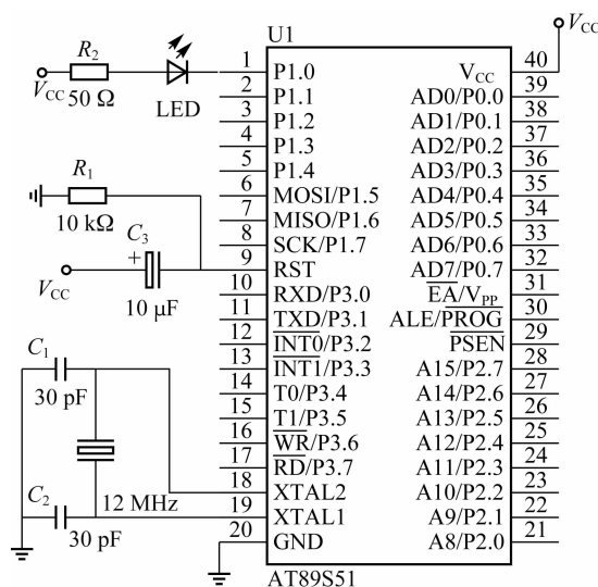
图 1-20 “眨眼”的 LED 电路原理图
