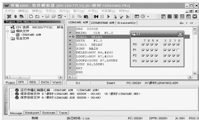
图 1-23 “眨眼”的 LED 程序仿真图(位操作)
