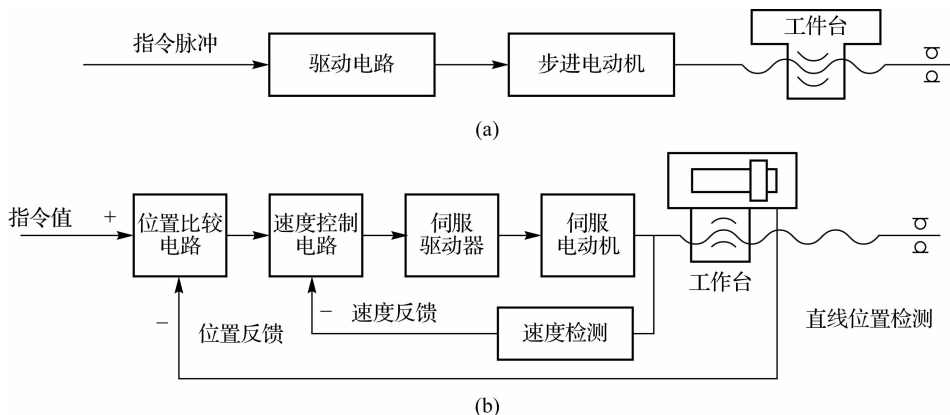
图 0-11 两种伺服系统的控制原理示意图
